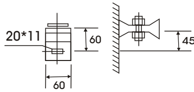
DUVAR TUTURMA KLİPSİ
