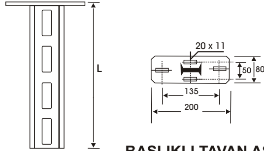
BAŞLIKLİ TAVAN ASKISI
